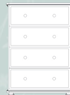
4 DRAWER JUMBO CHEST WTRD143 WPRM143 h:1145 w:810 d:495
