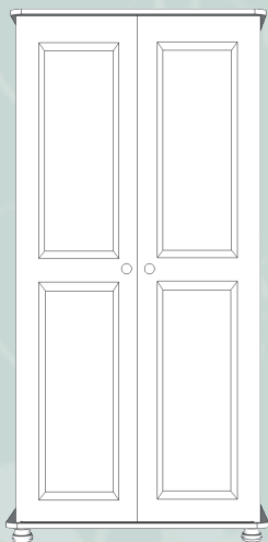
2 DOOR FULL LENGTH ROBE WTRD116 WPRM116 h:1870 w:915 d:545
